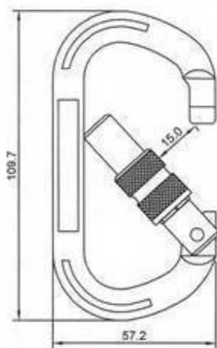
CONDIÇÃO ABERTA
