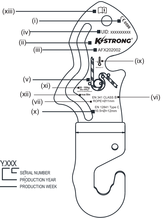
UPPER FLANGE
